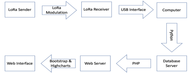
Fig. 1. LouPe system diagram
